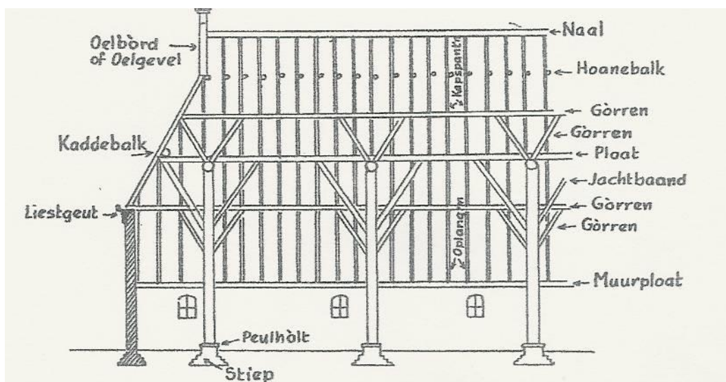
Fig. 75. Zijk-aanzicht van n goul, (dak weggedacht). Tekening van G. R. Jager.
